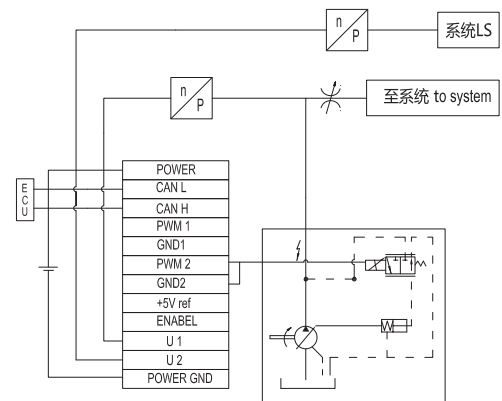
负载敏感变量泵
