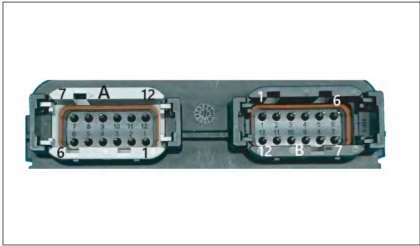
控制器端连接器 DTM13-12PA-12PB-R008
