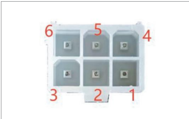
总线开关端针座 5569-6AW
