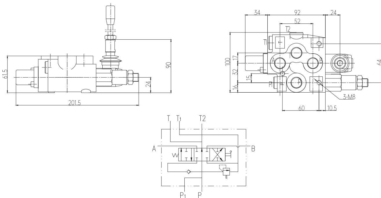
GDV25-1: 1联整体阀
