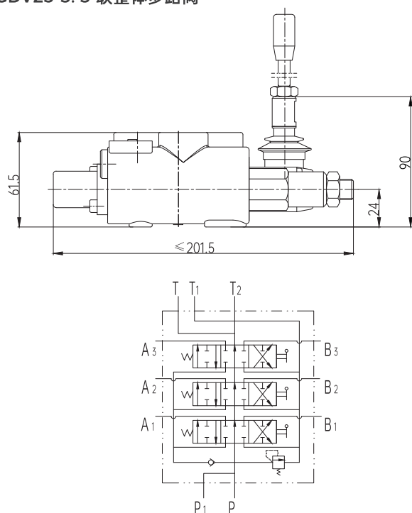
GDV25-3: 3 联整体多路阀
