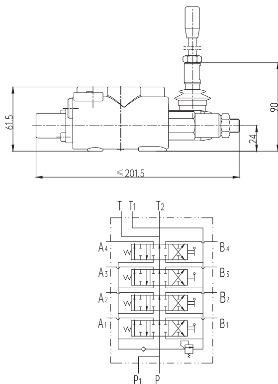
GDV25-4: 4 联整体多路阀
