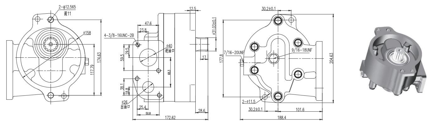
2P9239 Dimensions
